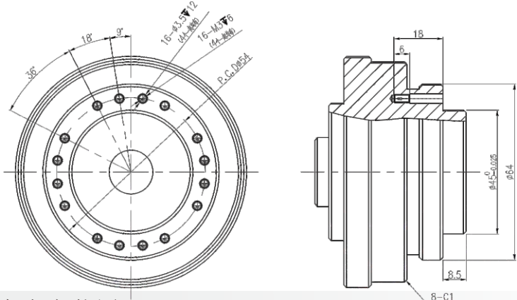
机械手底座安装图
