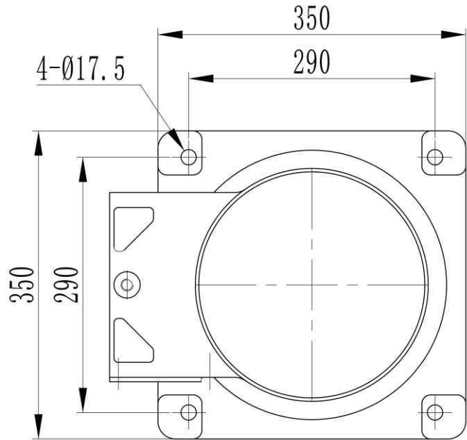
机械手底座安装图
