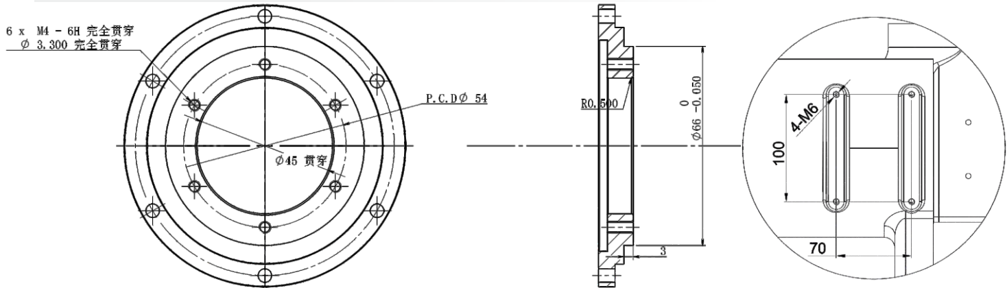
机械手底座安装图
