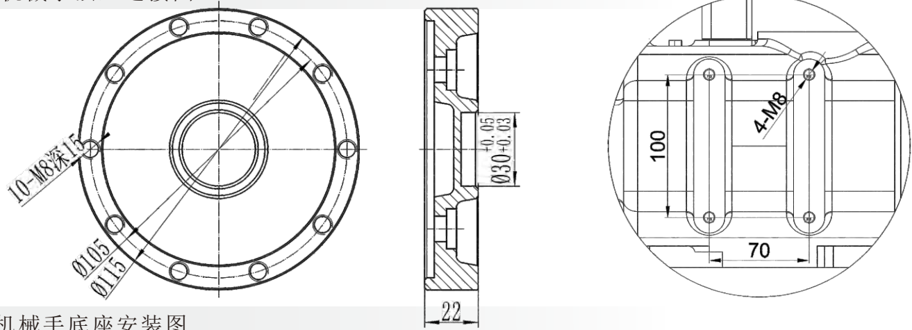
机械手底座安装图
