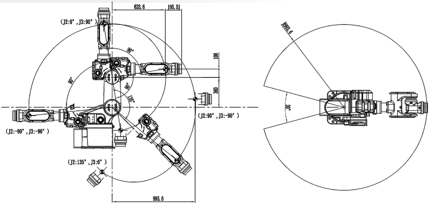
机械手法兰连接图
