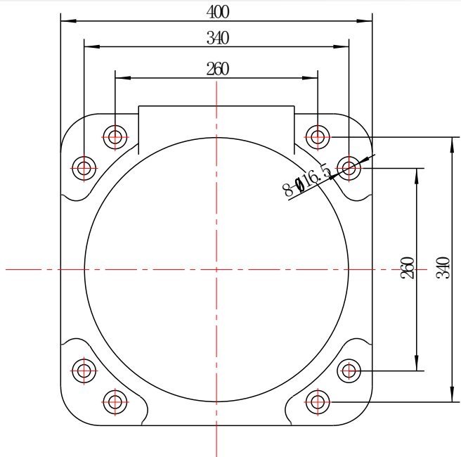
机械手底座安装图
