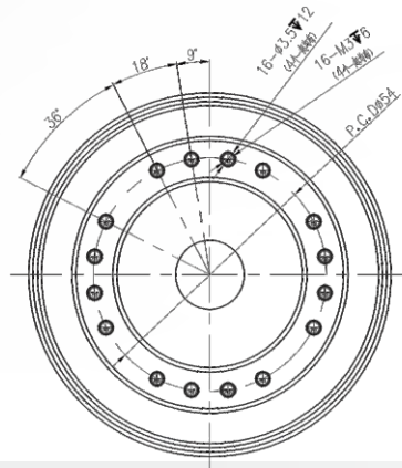
机械手底座安装图
