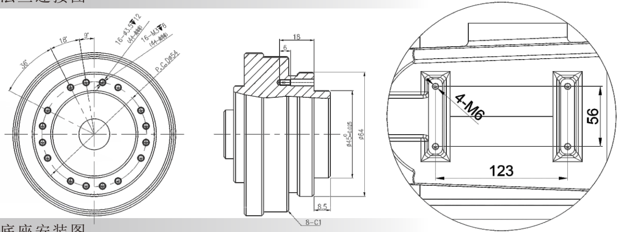
机械手底座安装图
