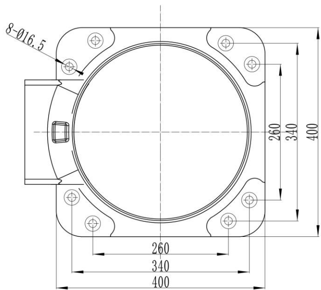
机械手底座安装图
