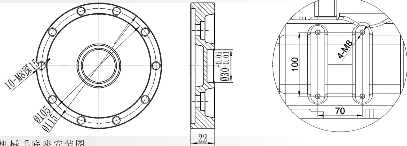
机械手底座安装图
